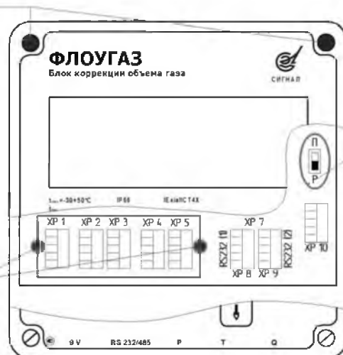
Рисунок 2. Схема пломбировки блока коррекции объема газа «ФЛОУГАЗ»
